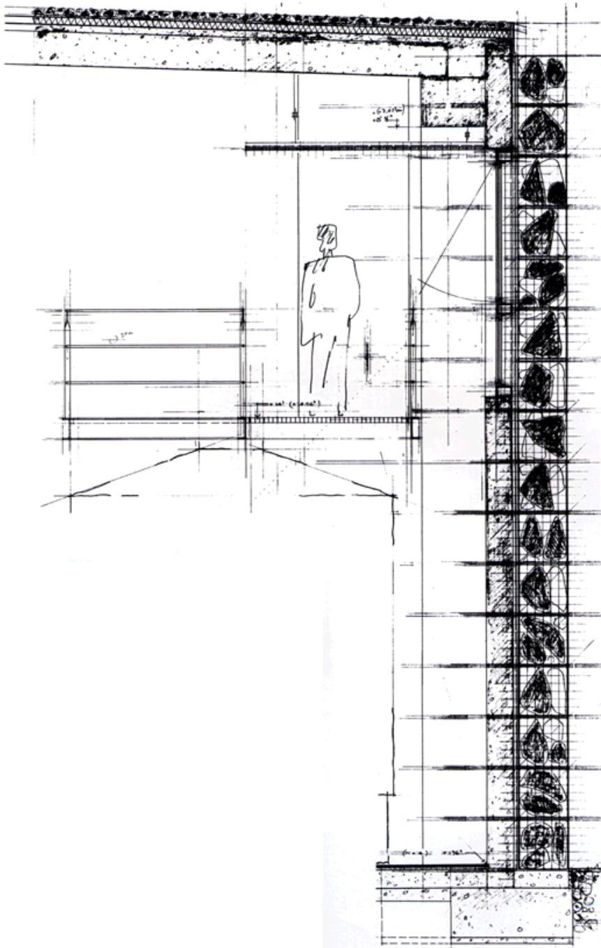
Sección vertical de cerramiento Vertical wall section
